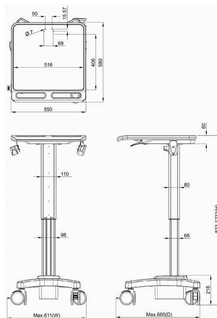
Målskisse (mm)
